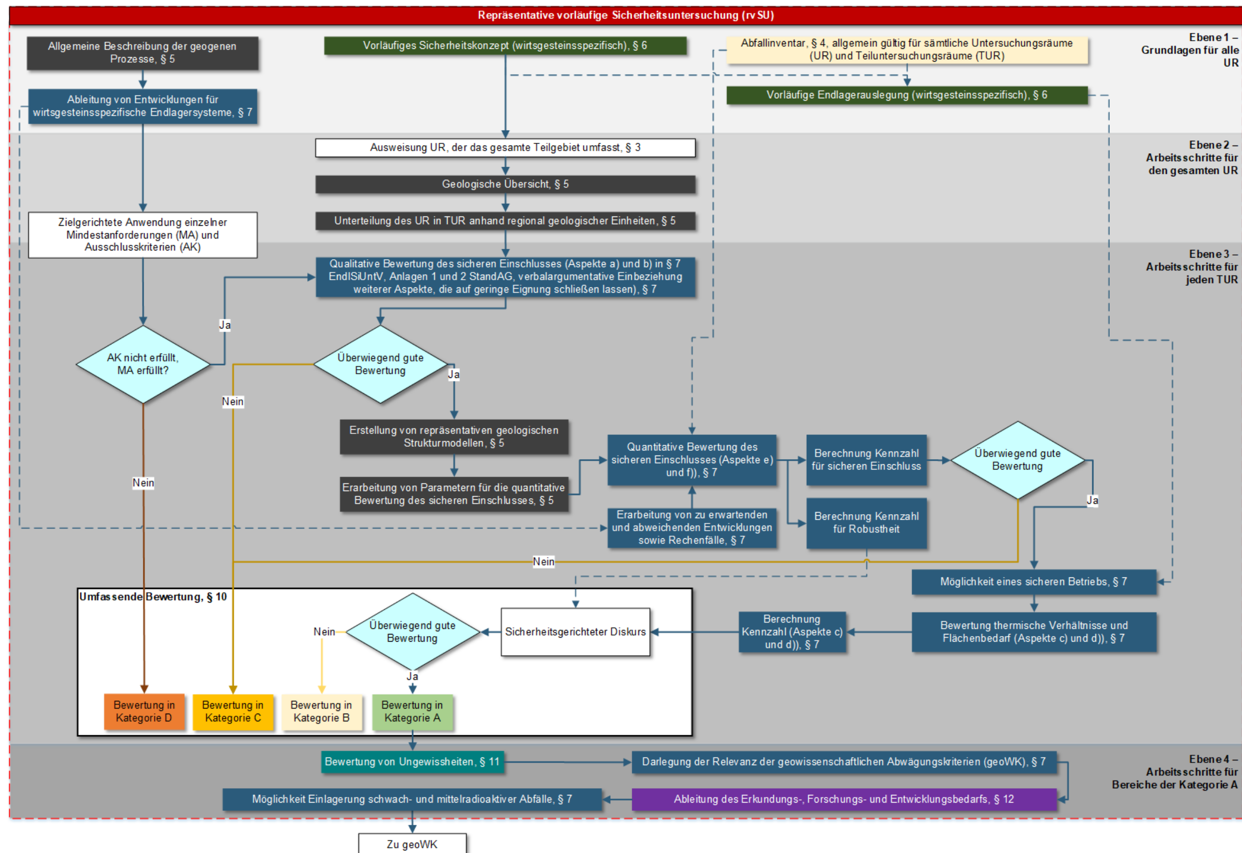
Abbildung 9: Ablauf der Bearbeitungsschritte einer rvSU.
